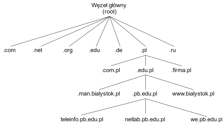
Rys. 1. Fragment hierarchii systemu DNS
